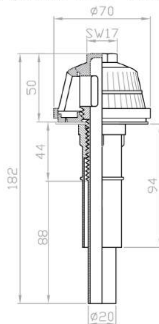
CHỤP LỌC CÁT CHÂN VỪA KHÔNG CÓ RĂNG GIÓ ( Sử dụng tán dài - đan bê tông )
