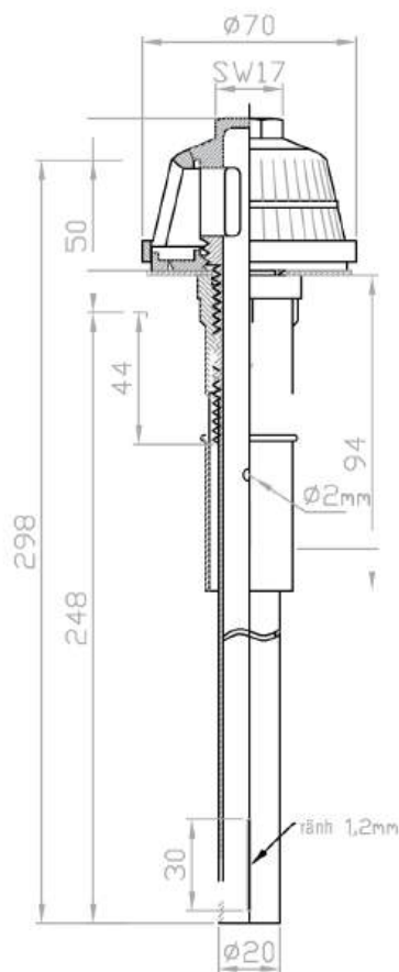
CHỤP LỌC CÁT CHÂN VỪA CÓ RĂNG GIÓ ( Sử dụng tán dài - đan bê tông )
