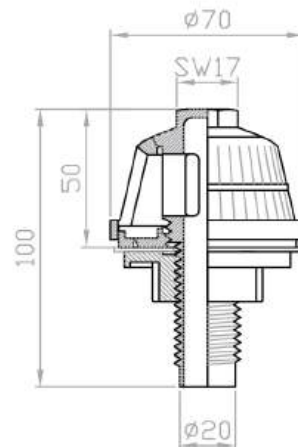
CHỤP LỌC CÁT CHÂN NGẮN KHÔNG CÓ RĂNG GIÓ ( Sử dụng tán ngắn - đan Inox )
