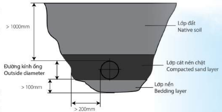
Minh họa: cách lắp đặt ống dưới mặt đất
