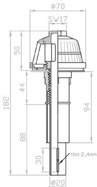
CHỤP LỌC CÁT CHÂN VỪA CÓ RĂNG GIÓ ( Sử dụng tán dài - đan bê tông )
